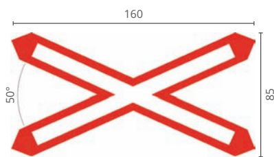
Figura II 10/a Art.87 CROCE DI S.ANDREA Segnala l'immediata vicinanza di un attraversamento ferroviario senza barriere ad 1 binario, ed indica l'obbligo di fermarsi in corrispondenza della striscia di arresto.
