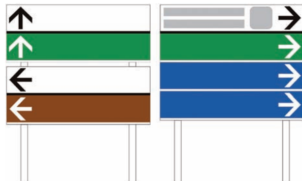
Figura II 255 Art.128 GRUPPO SEGNALETICO UNITARIO URBANO BIFILARE Se i segnali di direzione sono in numero eccessivo conviene sempre frazionarli in gruppi più piccoli con frecce omogeneamente dirette verso la stessa direzione e disposti in posizione contigua o nei punti più appropriati della intersezione.
