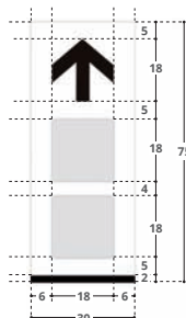
Figura II 288 Art.132 SEGNALE DI CONFERMA URBANO Conferma la direzione verso punti di interesse pubblico urbano.
