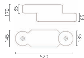
Figura 483 CORDOLO JOLLY Cordolo realizzato in plastica riciclata, ideale per la realizzazione di rotatorie di qualsiasi diametro, cordolature per marciapiedi, aiuole e isole spartitraffico. Atti a sostituire i cordoli in cemento, attenuano l'urto in caso di incidente per una maggior sicurezza. 1 m lineare = 2,5 pezzi. Dimensioni: 52x14,5x17 cm Disponibile: - giallo - bianco - nero
