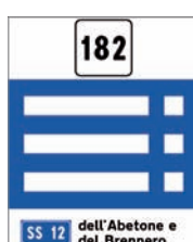
Figura Il 265 Art.129 PROGRESSIVA DISTANZIOMETRICA INTEGRATA CON SEGNALE DI CON- FERMA SU STRADE EXTRAURBANE
